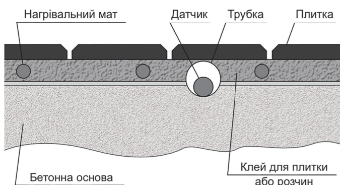
Розріз підлоги мат EASYTHERM EM
