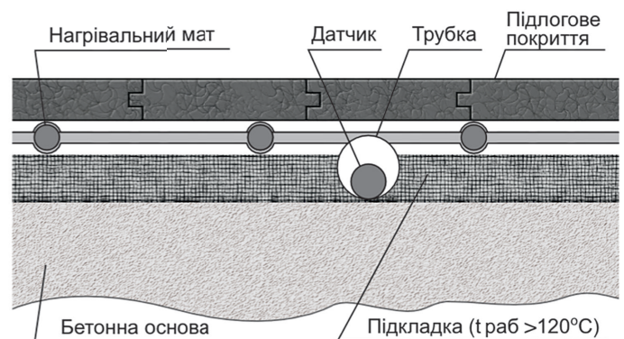
Розріз підлоги мат EASYTHERM EMF
